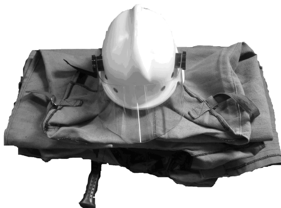
Рисунок 1 (г) – Укладання бойового одягу та спорядження першим способом (загальний вигляд укладеного бокового одягу та спорядження)
