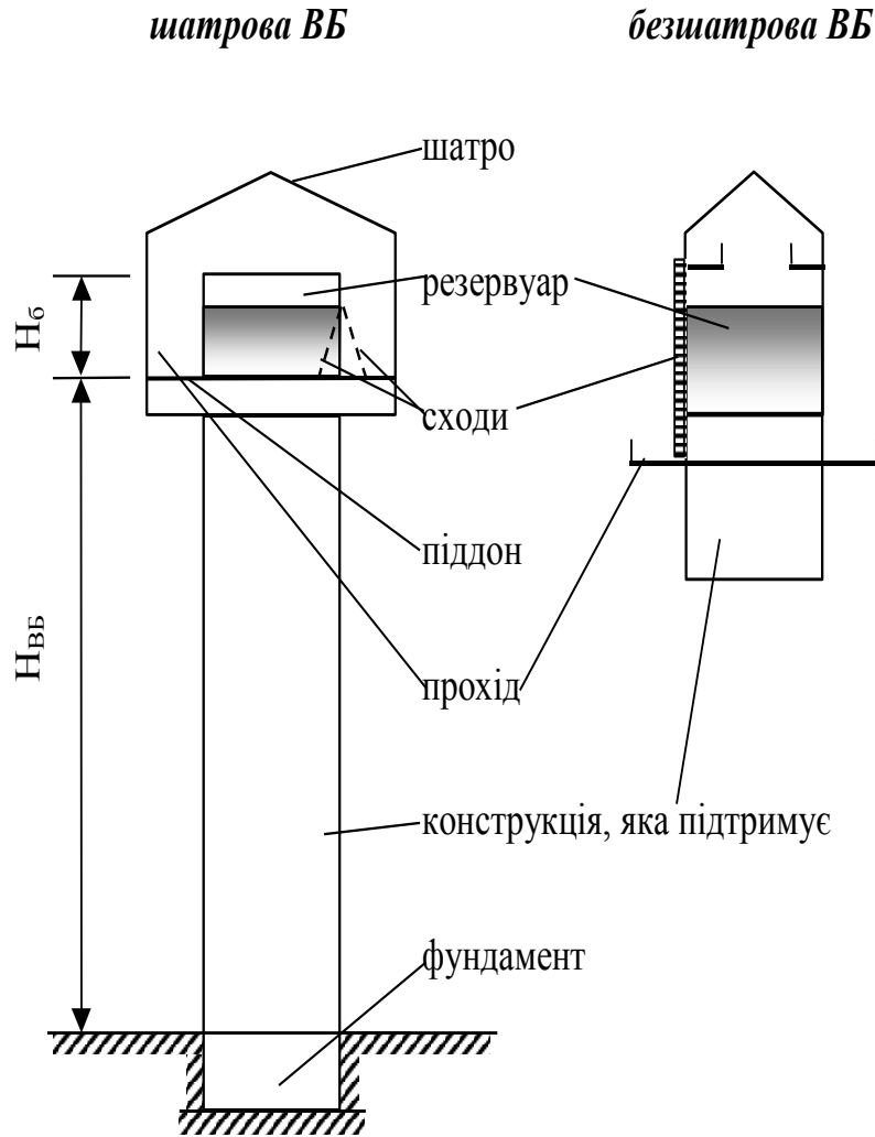
Рис.6.3 – Конструктивні складові водонапірних башт
