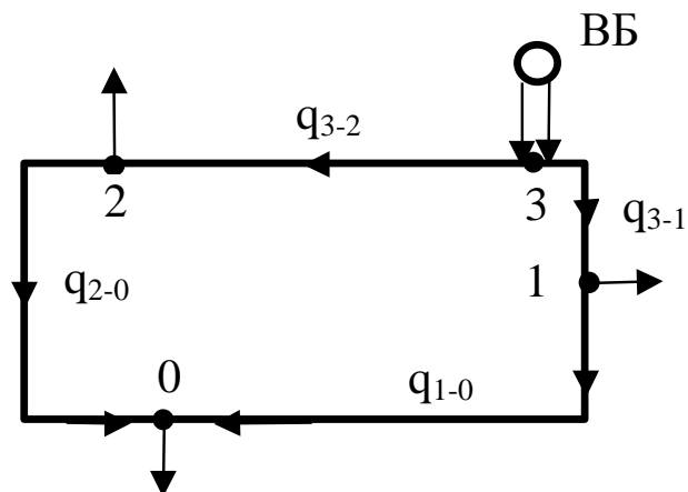
Рис.4.2 – Розрахункова схема кільцевої водопровідної мережі: 0-3 – точки відбору води
