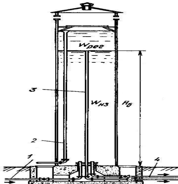
Рис.6.7 - Гідроколони:
