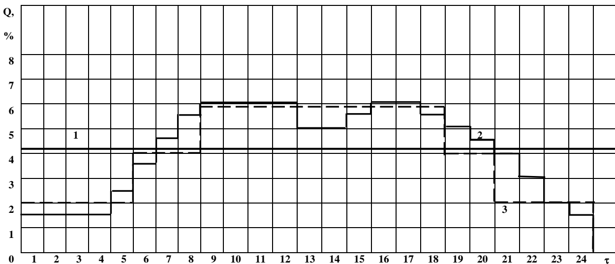
Рис.3.1 - Графік водоспоживання:
