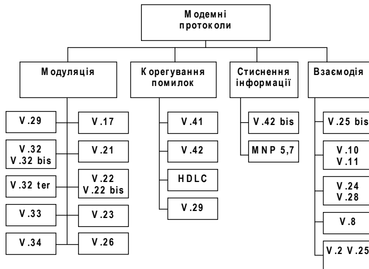
Рис. 5.5 – Модемні протоколи
