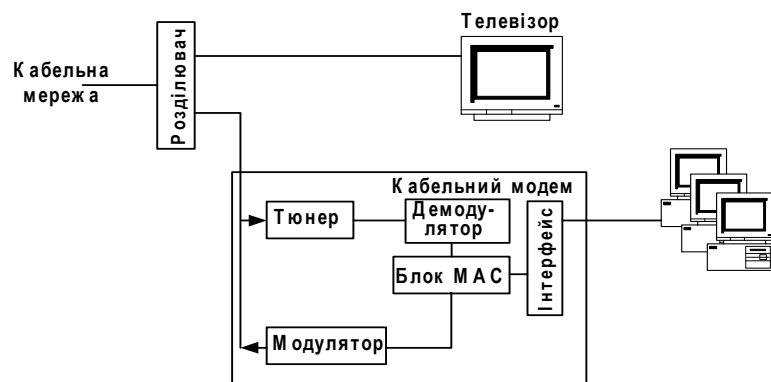
Рис. 5.6 – Структурна схема кабельного модему
