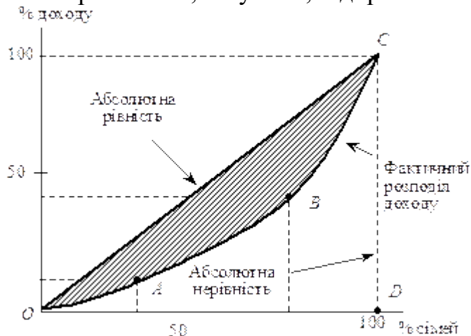
Рис.1. Крива Лоренца
