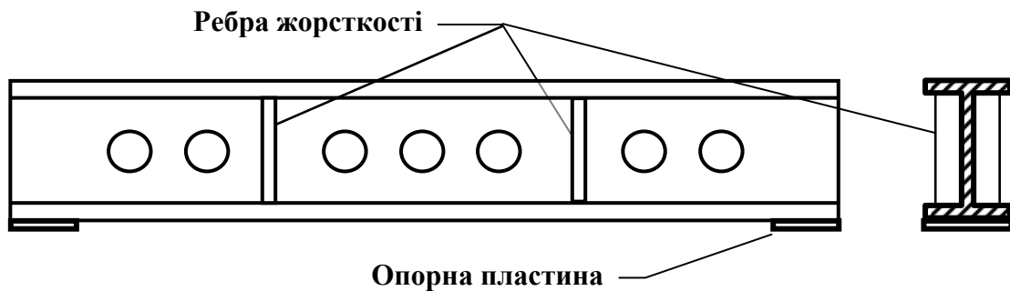
Рисунок 4.22 – Будова сталевої кроквяної балки покриття
