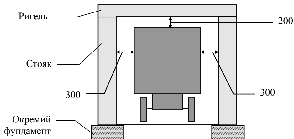
Рисунок 4.20 – Схеми просвітів у воротах
