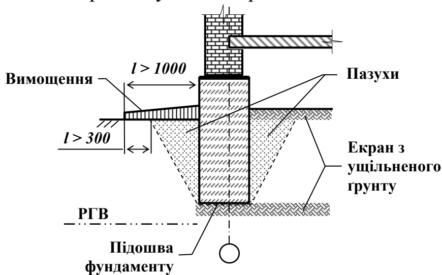
Рисунок 5.5 – Приклад застосування заходів для захисту фундаментів від замочування
