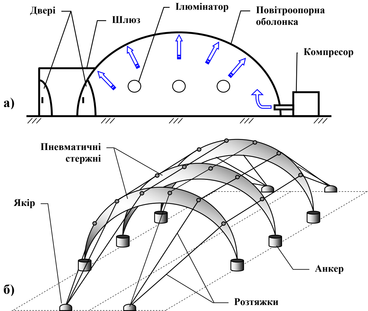
Рисунок 6.10 – Пневматичні покриття:
