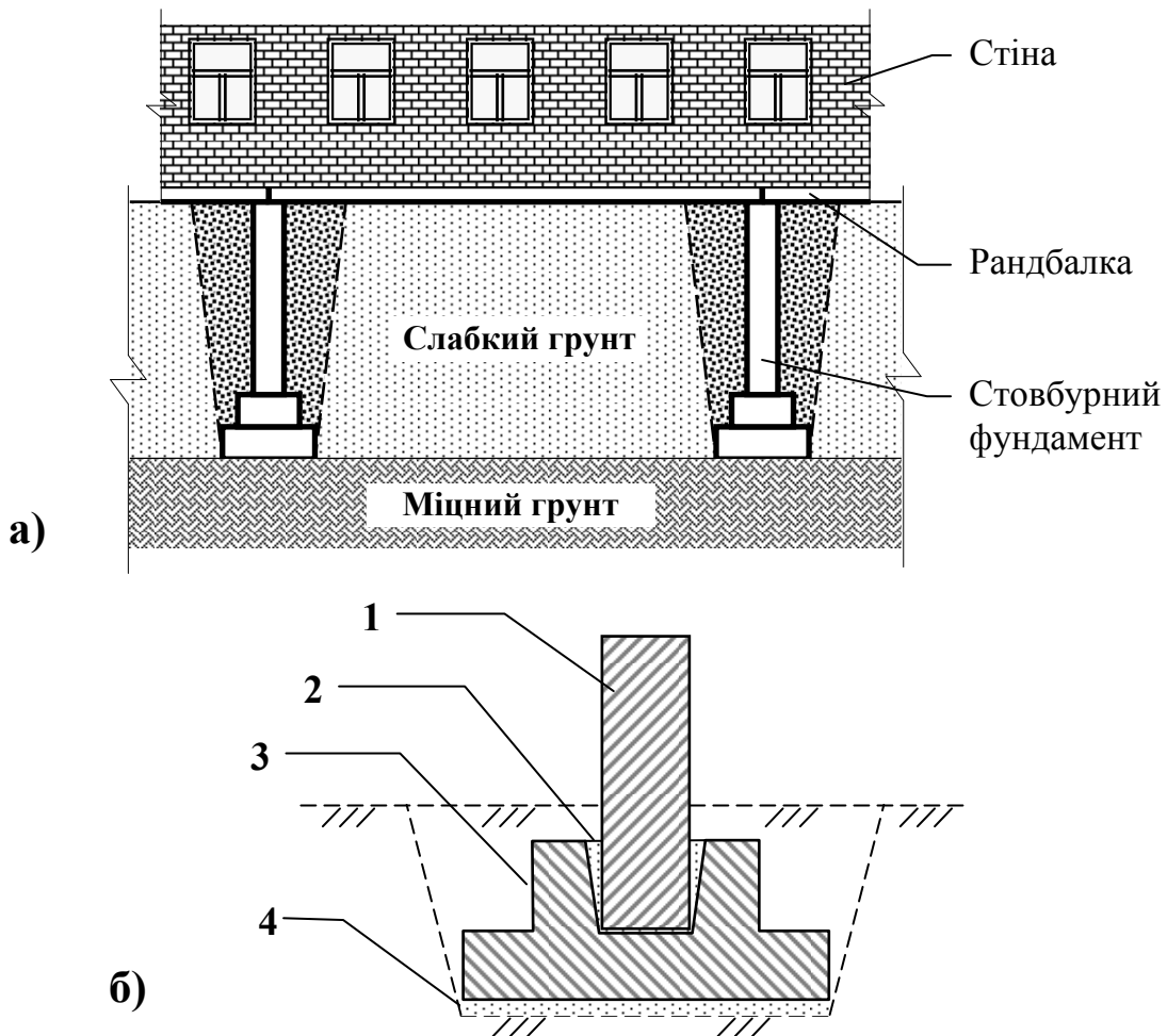
Рисунок 3.4 – Приклад конструкції стовбурних фундаментів: звичайного (а) та стаканного (б) типу:
