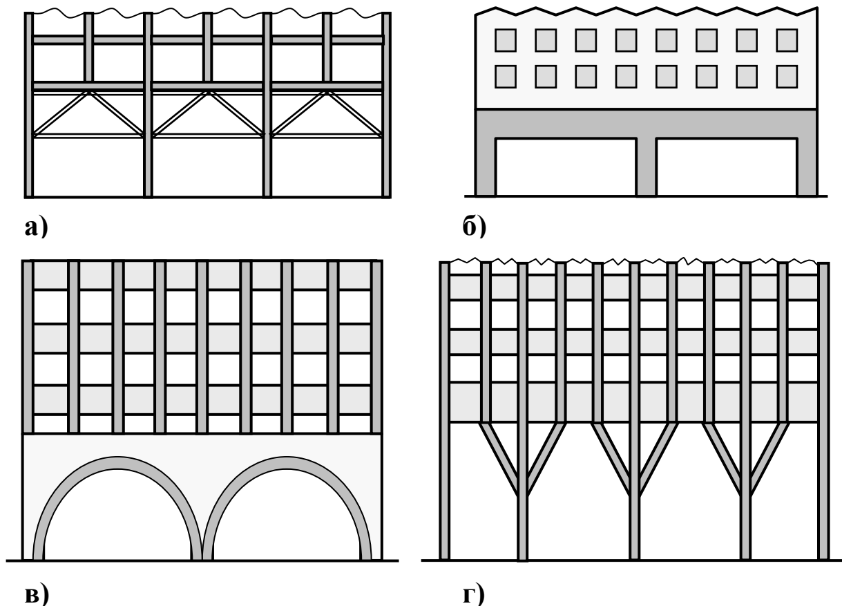
Рисунок 6.18 – Варіанти конструктивних рішень першого поверху будівель підвищеної поверховості: а) розкісна ферма; б) балка-стіна; в) багатопрольотна арка; г) об'єднання груп стояків (стрільчаті арки)
