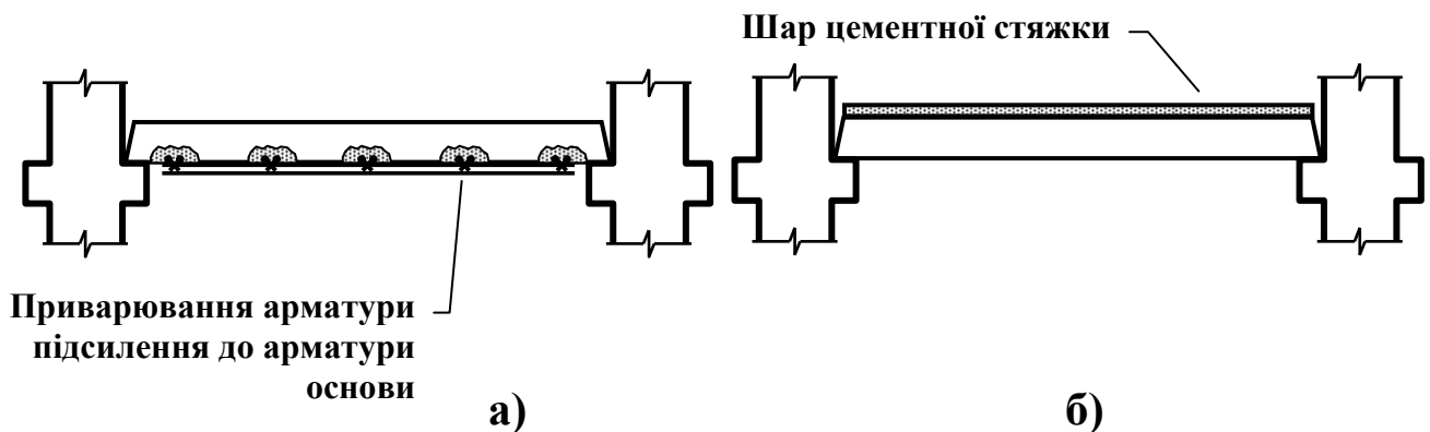
Рисунок 6.24 – Підсилення залізобетонних плит нарощуванням перетину: а) у зоні розтягнення; б) у зоні стиску
