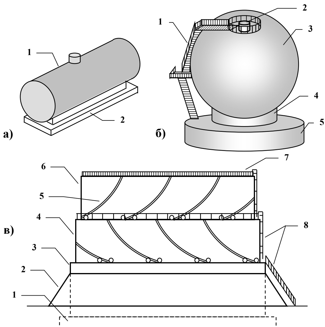
Рисунок 4.36 – Газгольдері:
