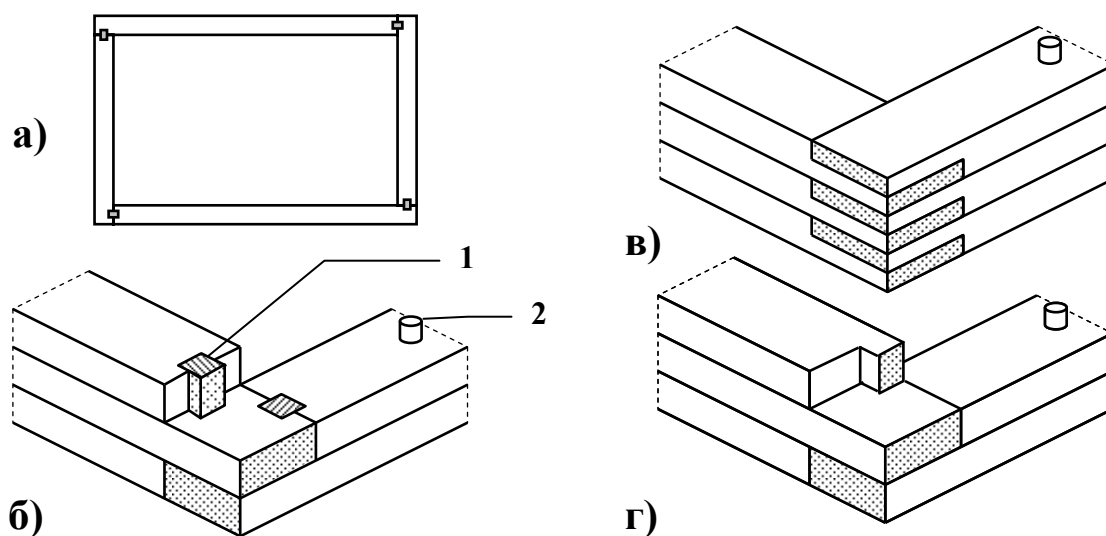
Рисунок 3.11 – Приклади з'єднання брусів брусчатої стіни:
