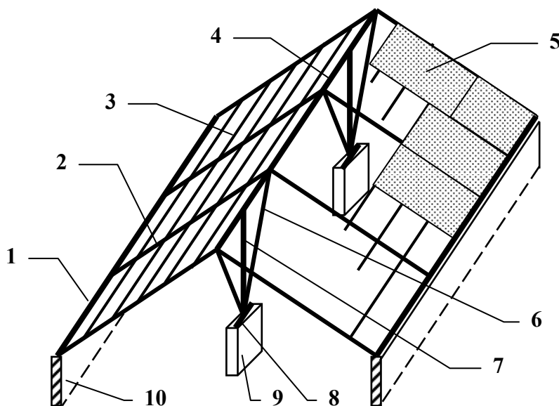
Рисунок 3.22– Схема розташування конструкцій приставного схильного даху:
