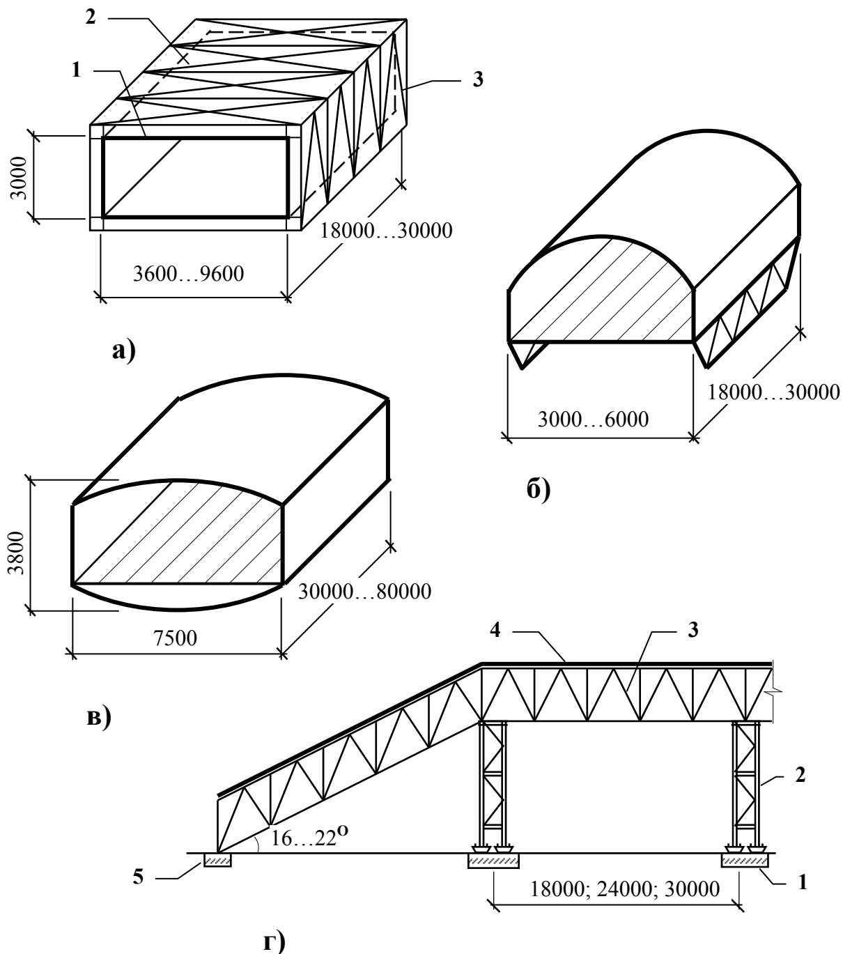
Рисунок 4.38 – Галереї:
