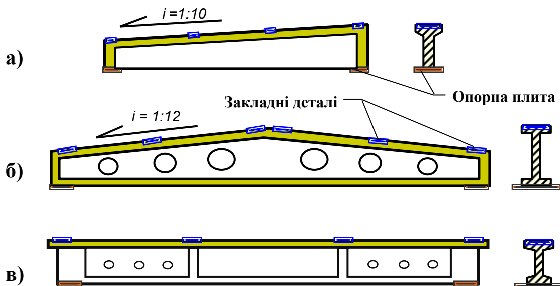
Рисунок 4.21 – Види залізобетонних кроквяних балок покриття: а) односхильна; б) двосхильна; в) з паралельними поясами
