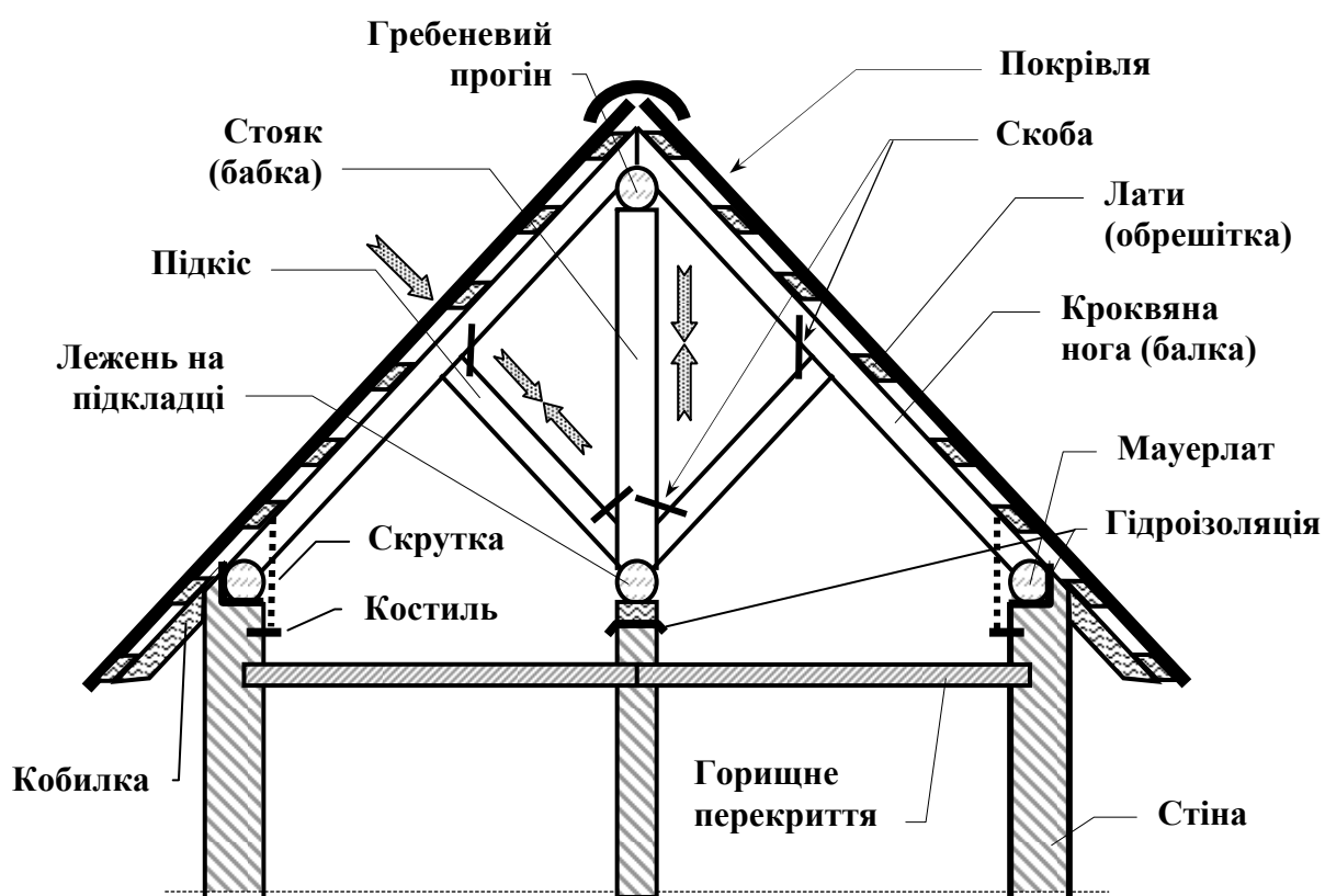
Рисунок 3.23 – Конструкція схилого приставного даху
