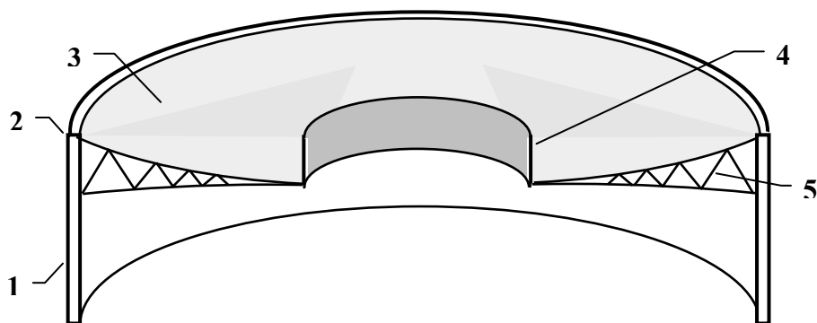
Рисунок 6.7 – Мембранне покриття:
