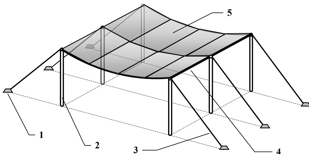
Рисунок 6.6 – Вантове покриття:
