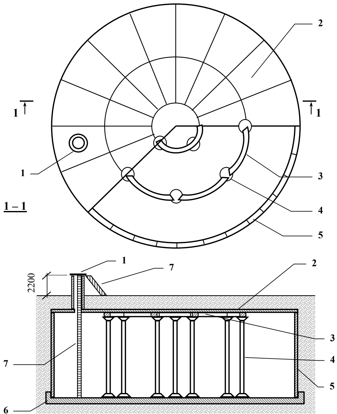
Рисунок 4.35 – Залізобетонний збірний підземний резервуар:
