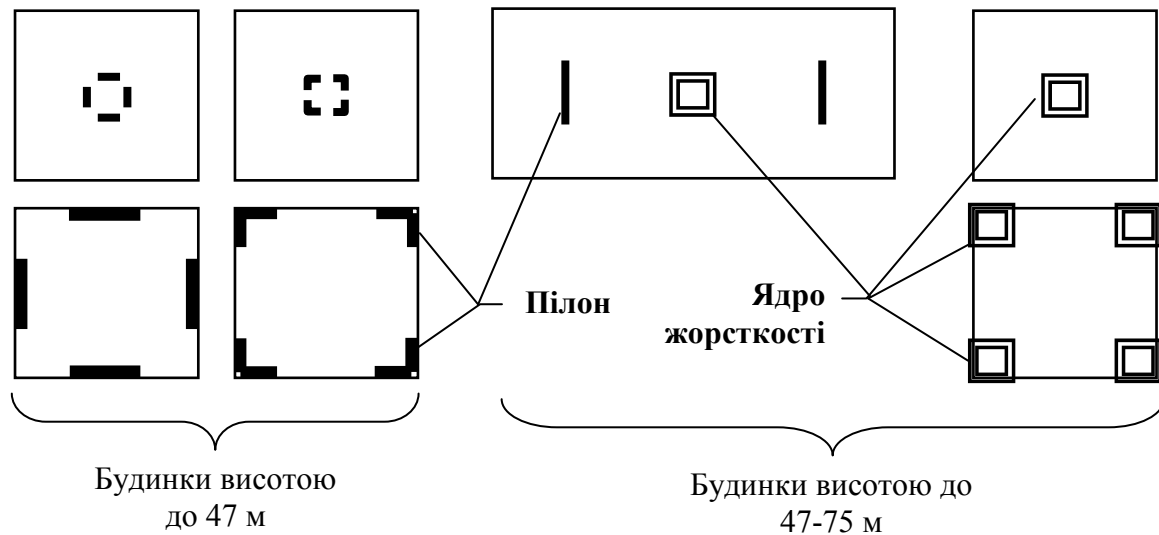
Рисунок 6.15 – Характерне розташування пілонів та ядер жорсткості в будівлях підвищеної поверховості та висотних
