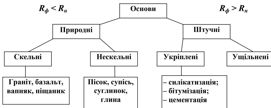
Рисунок 3.1 – Основи фундаментів
