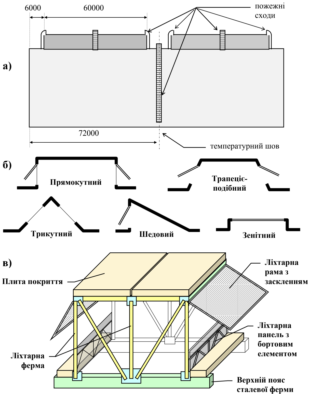
Рисунок 4.31 – Ліхтарні конструкції
