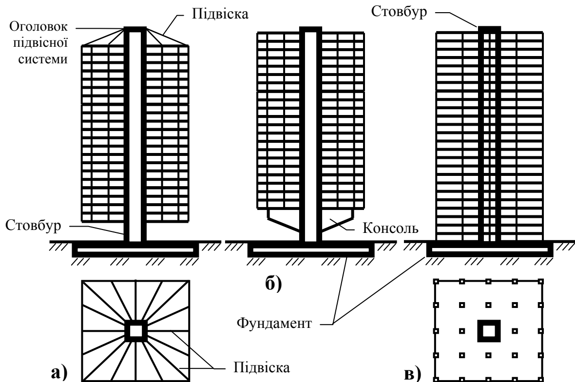
Рисунок 6.16 – Схеми будівель підвищеної поверховості стовбурної системи:
