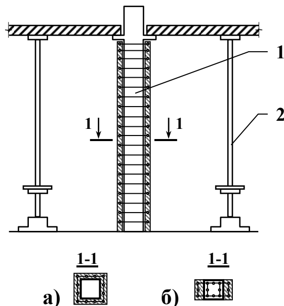
Рисунок 6.21 – Підсилення залізобетонної колони методами: а) встановлення обойми; б) нарощуванням перетину 1 – колона; 2 – домкрат
