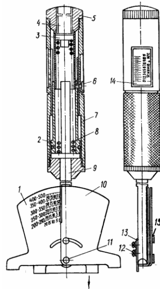
Рис. 2.10. Пристосування КИ-8920 для перевірки натягу паса:
