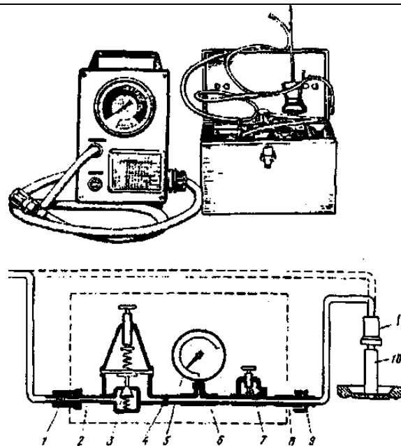
Рис. 1.7. Прилад К-69М
