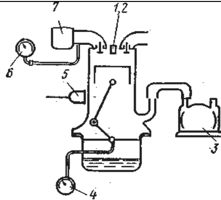
Рис. 1.1 Схема діагностування бензинового двигуна:
