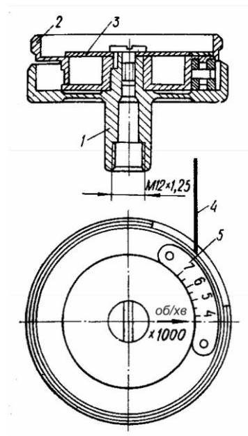
Рис. 2.8. Прилад КИ-1308В для вимірювання частоти обертання ротора масляної центрифуги: 1 – корпус; 2 – маховичок; 3 – індекс; 4 – язичок; 5 – шкала.
