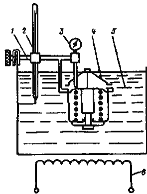
Рисунок 2.3. Схема приладу для перевірки термостата: 1 - кронштейн для кріплення термостата; 2 - тер-
