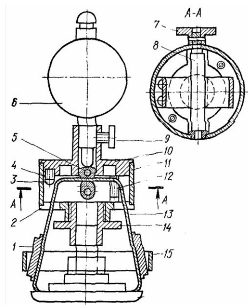
Рис.2.9. Пристосування КИ-9912 для визначення ступеню забрудненості роторів центрифуг:
