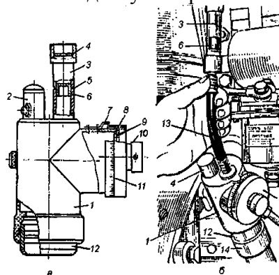
Рис. 1.9 Індикатор витрати газів КІ-13671-ГОСНИТІ: а – зовнішній вигляд; б – установка індикатора
