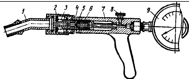
Рис. 1.17. Вакуум-аналізатор КИ-5315-ГОСНІТІ:
