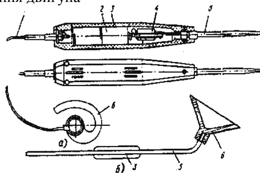
Рис. 1.3 Стетоскопи: а - електронний стетоскоп «Екранас»; б – стетоскоп мод. КИ-1154; 7 - дріт; 2 – елементи живлення; 3 - корпус-ручка; 4 - перетворювач віброударних імпульсів; 5 – звукочутливий стрижень; 6 - телефон-навушник
